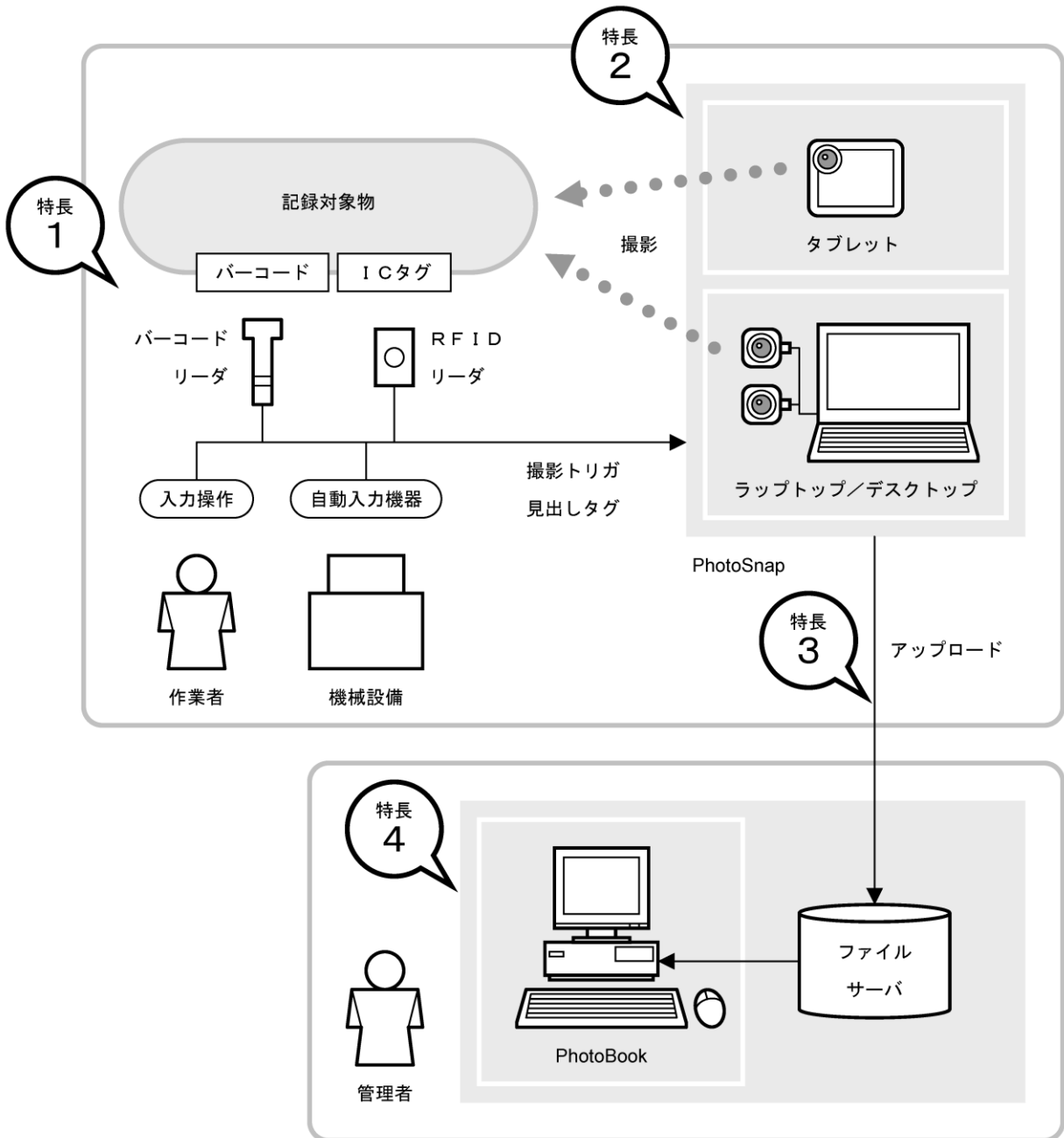
図. 「PhotoSnap」のシステム構成
